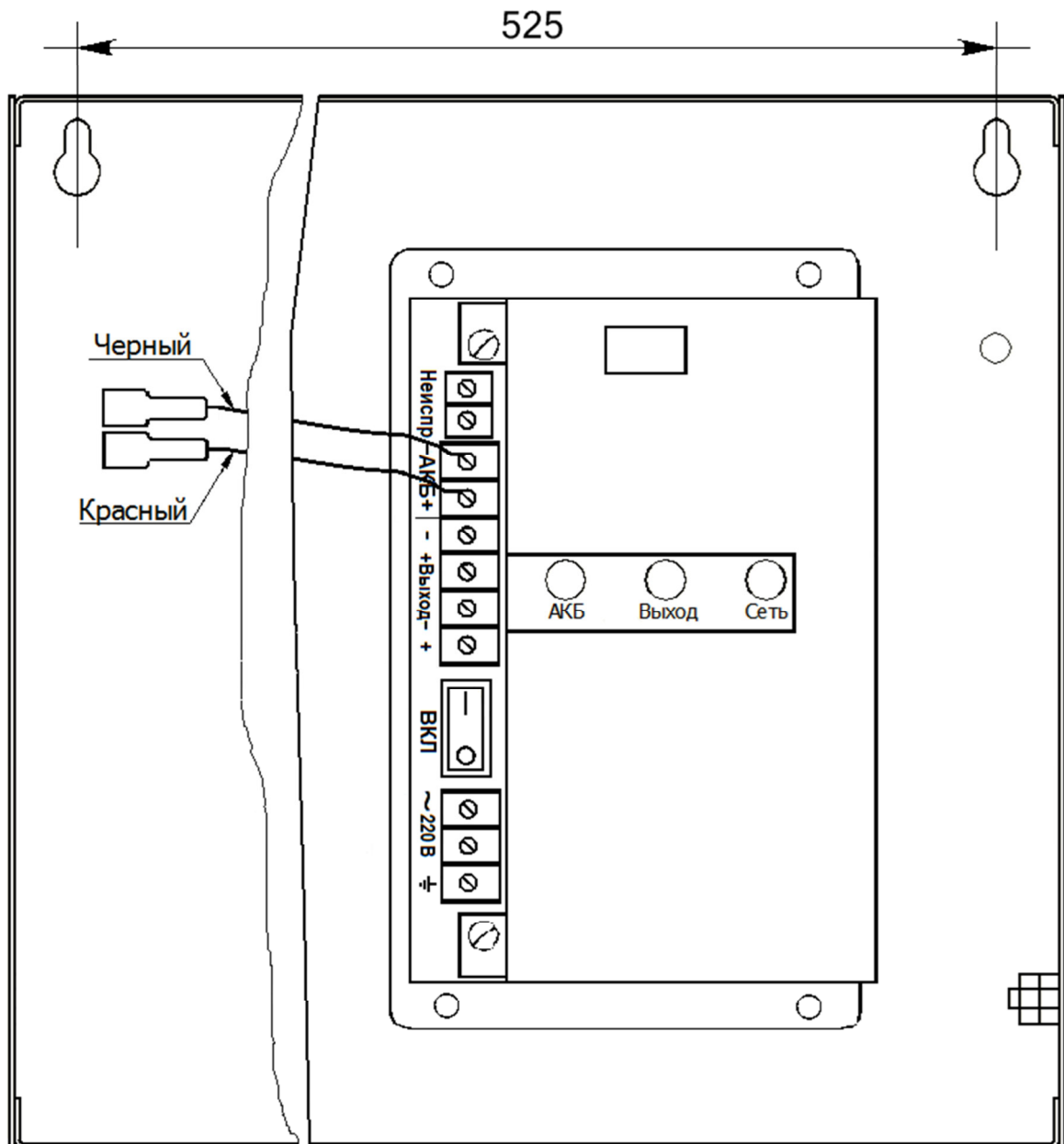
Рисунок 1 - Общий вид БРП со снятой крышкой
